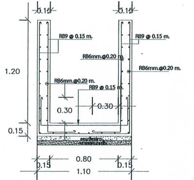
รูปตัด A
